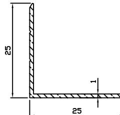
9554 0.131 kg/m
