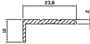
9051 0.148 kg/m
