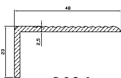
9026 0.430 kg/m
