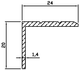
9050 0.192 kg/m
