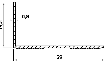
9587 0.134 kg/m
