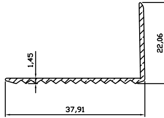
9361 0.165 kg/m
